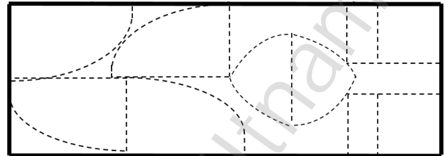
Polikarbonato lapo (6,0 x 2,1 m) pjaustymo schema šiltnamio galams uždengti
